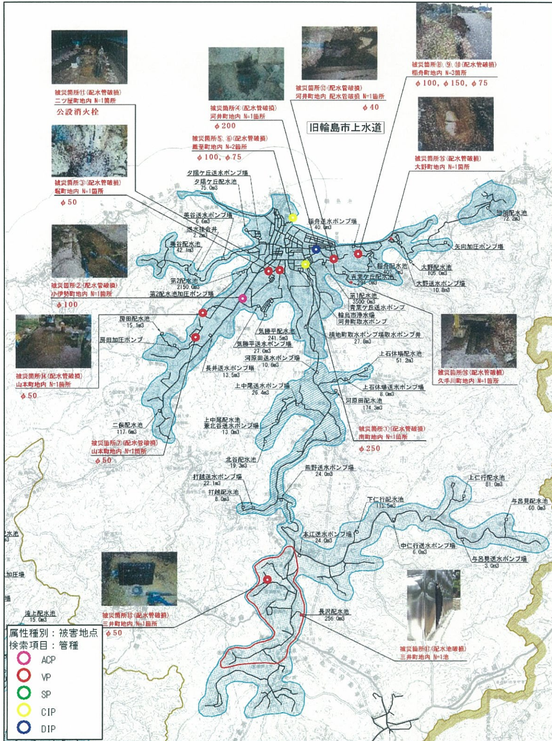
図 4.8 導・送・配水管の被害地点プロット図 (旧輪島市)
