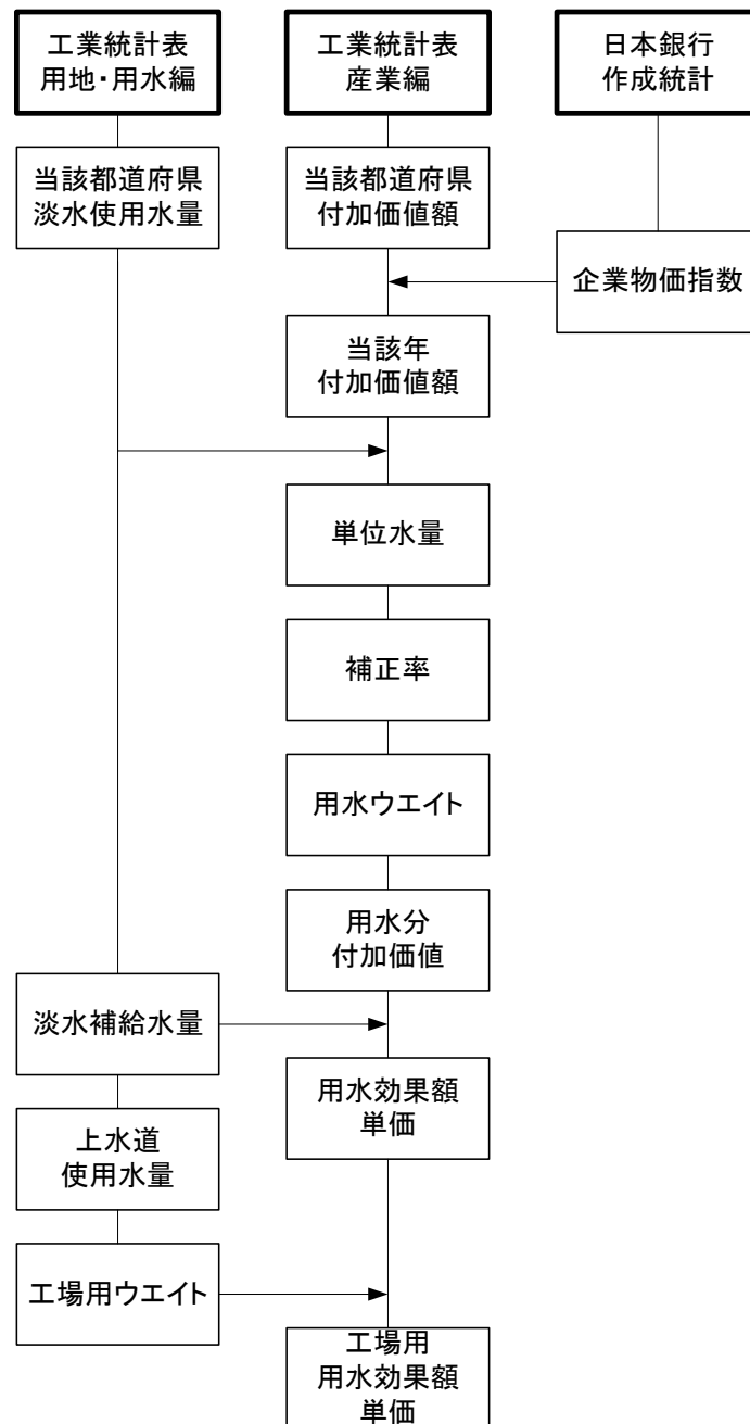
図V-3-5-1 用水効果額単価の算定方法
