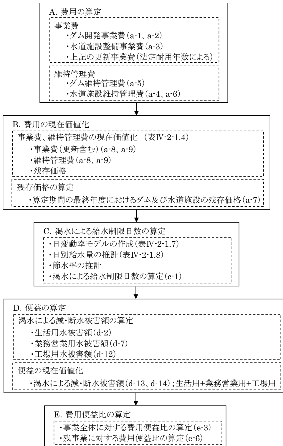
図IV-2-1.2 費用便益比の算定フロー
