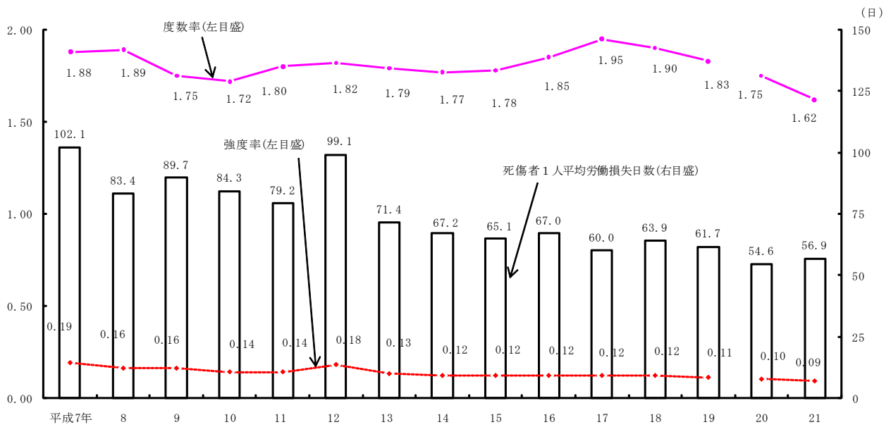
第1-1図 労働災害率及び死傷者1人平均労働損失日数の推移 〔調査産業計（総合工事業を除く）〕
