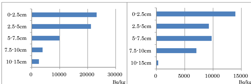
土壤の層別セシウム濃度
