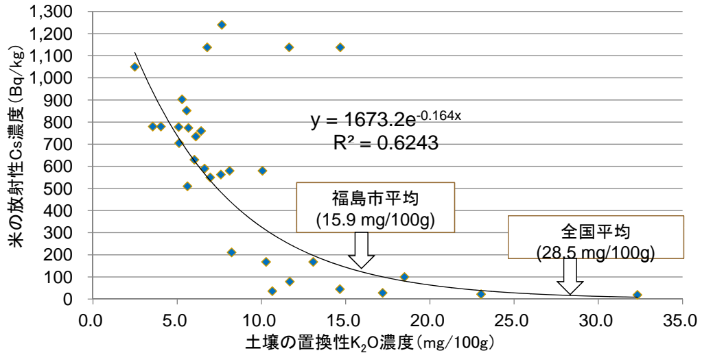
図 土壤の置換性カリウム濃度と玄米の放射性セシウム濃度との関係
