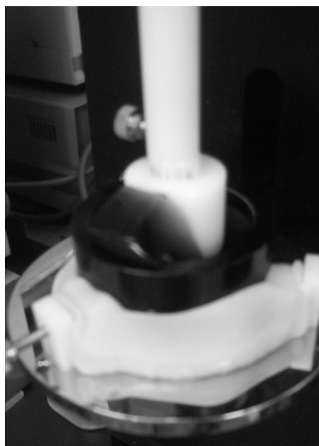
図3 高齢者用プランジャーによる測定
