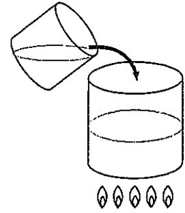
精製水とNaOHを加えアルカリ性下で1~2時間煮沸する
