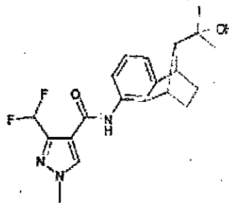
代謝物 Fa
