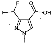
化合物 W
