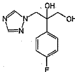
代謝物F
