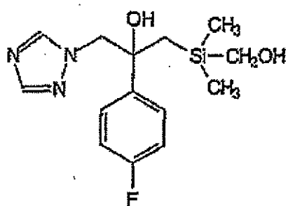
代謝物D
