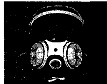
図4 半面形防じんマスクの例
