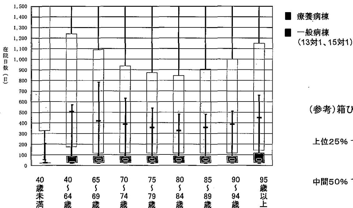
在院日数と年齢のクロス集計(箱ひげ図)
