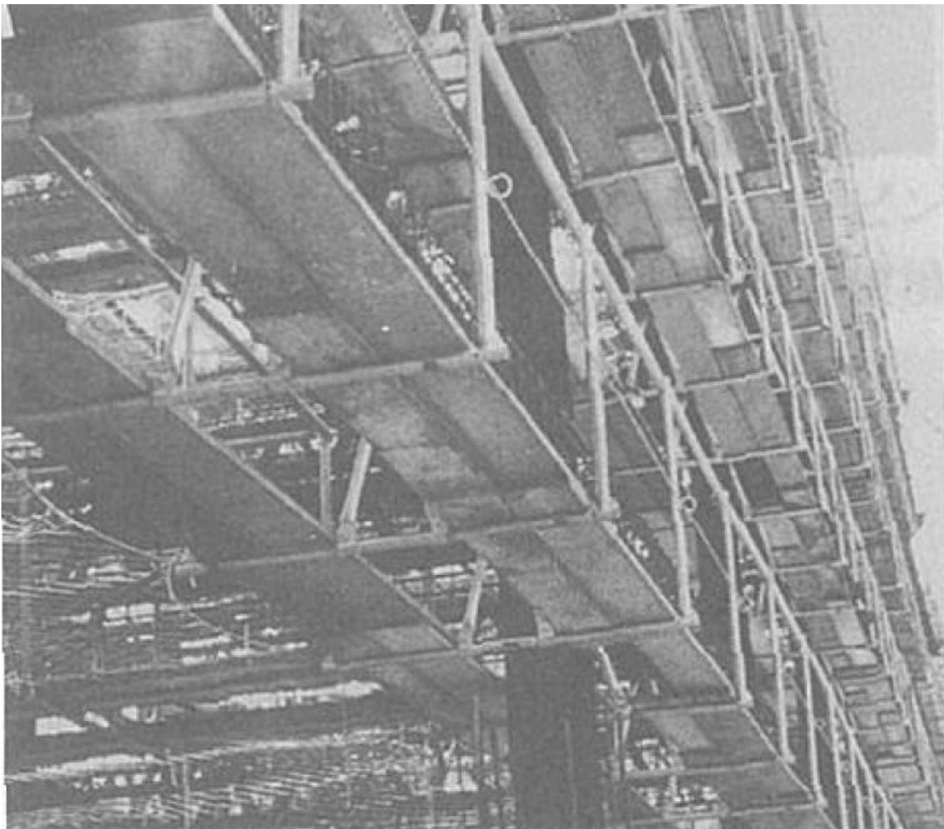
つり足場の例
