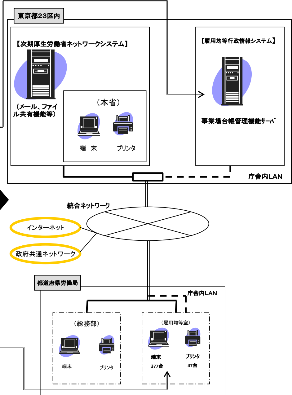
(次期)雇用均等行政情報システム構成図
