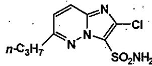
代謝物P
