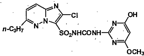
代謝物B
