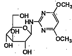
代謝物W
