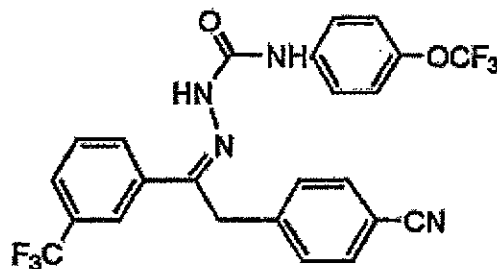
( Z -異性体)
