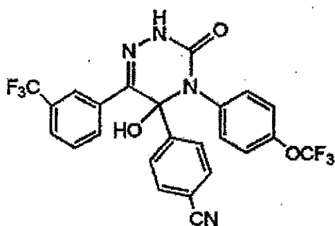
(代謝物C)
