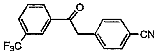
(代謝物D)
