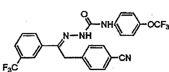
( E -異性体)
