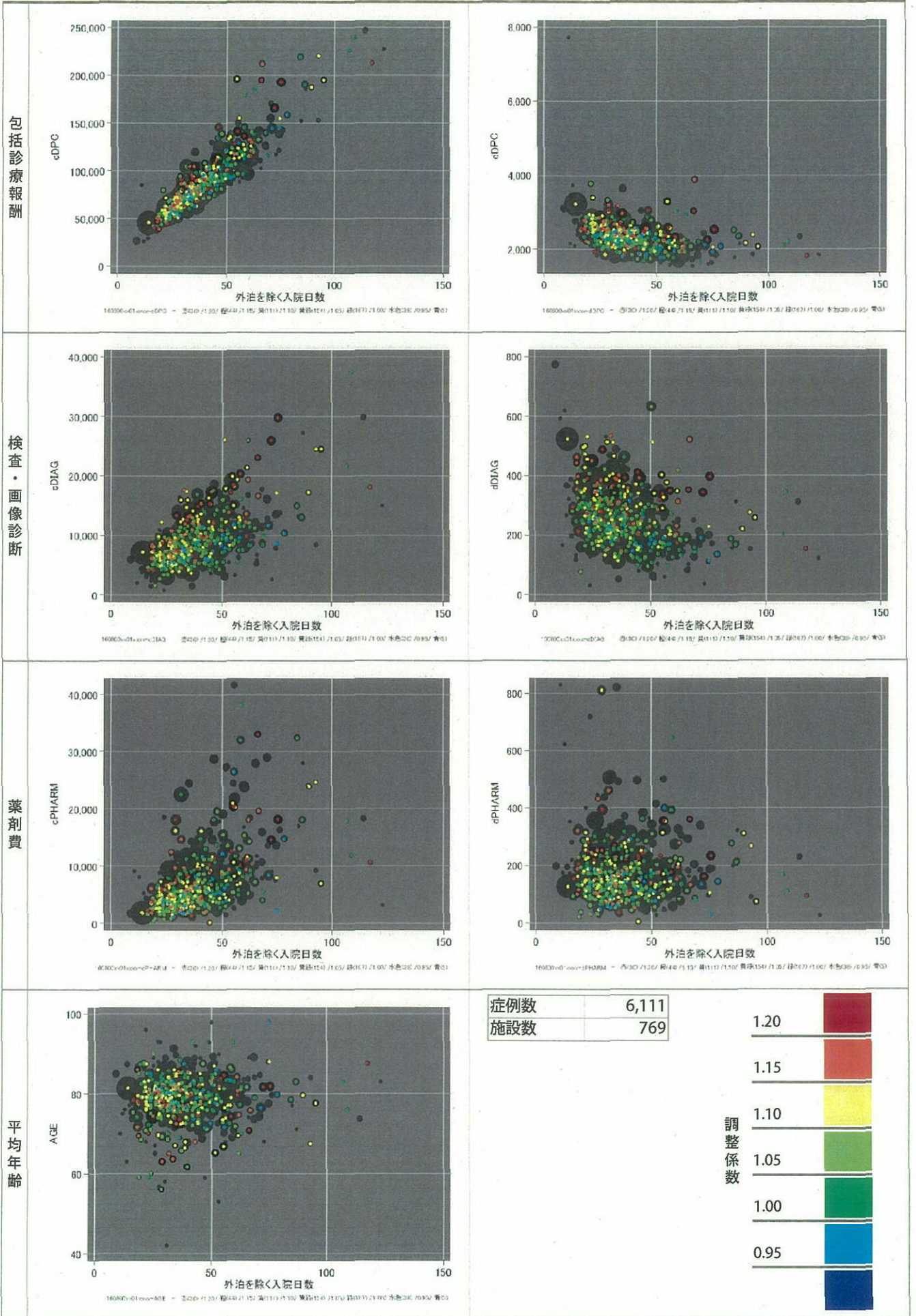
調整係数とデータのばらつきとの関係
