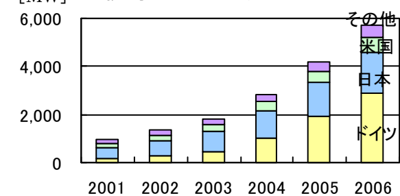
[MW] 累積導入量は世界トップレベル
