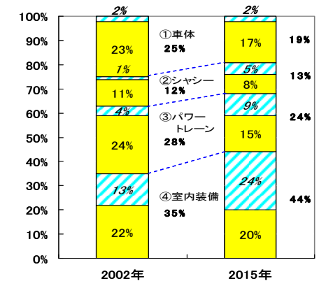
【自動車のコスト構造変化と拡大するエレクトロニクス・ソフトウェアの割合】
