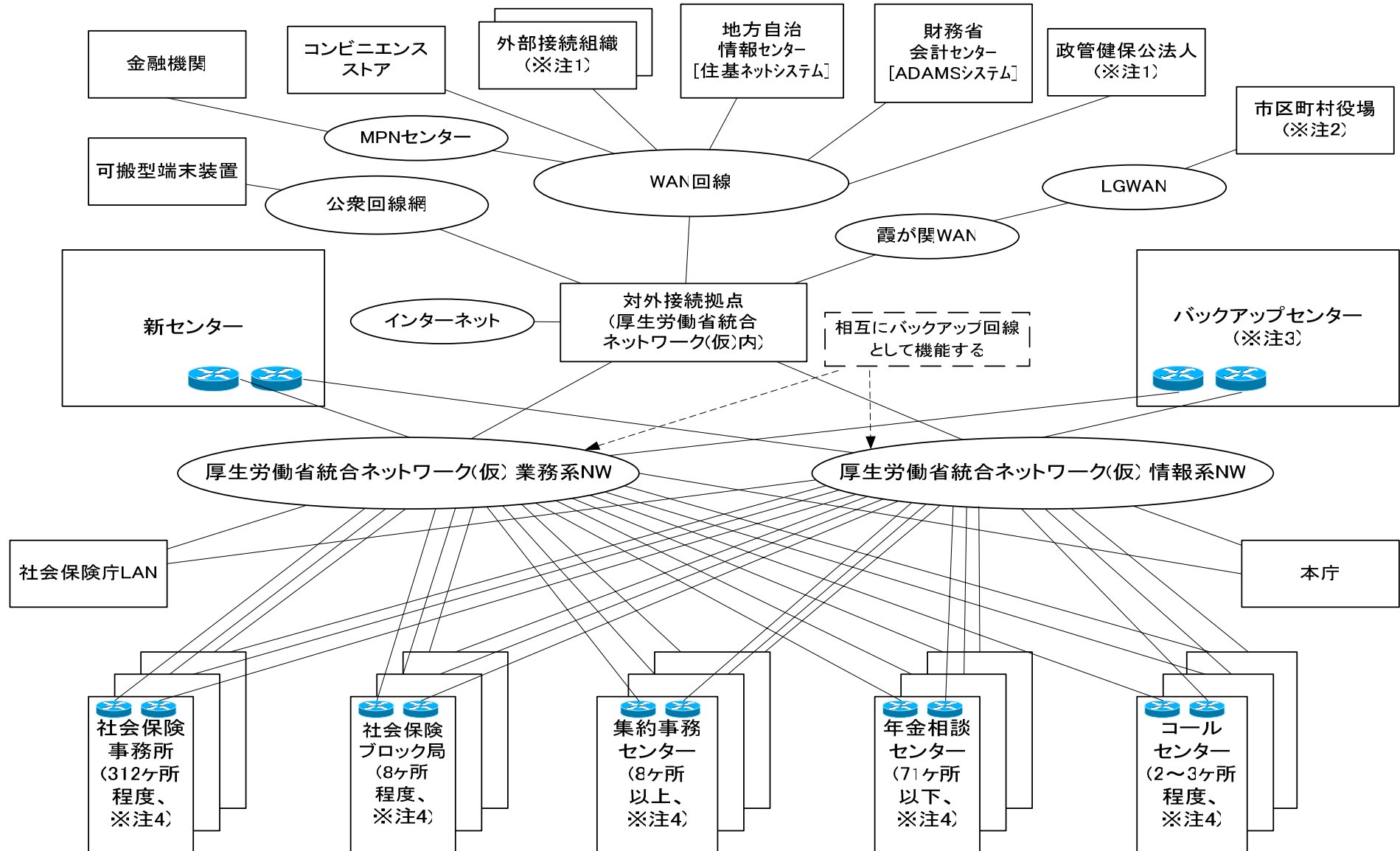
図1.ネットワーク構成図
