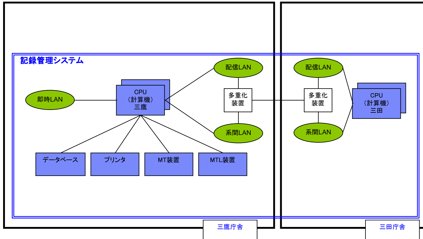
図2 ネットワーク構成図(記録管理システム)
