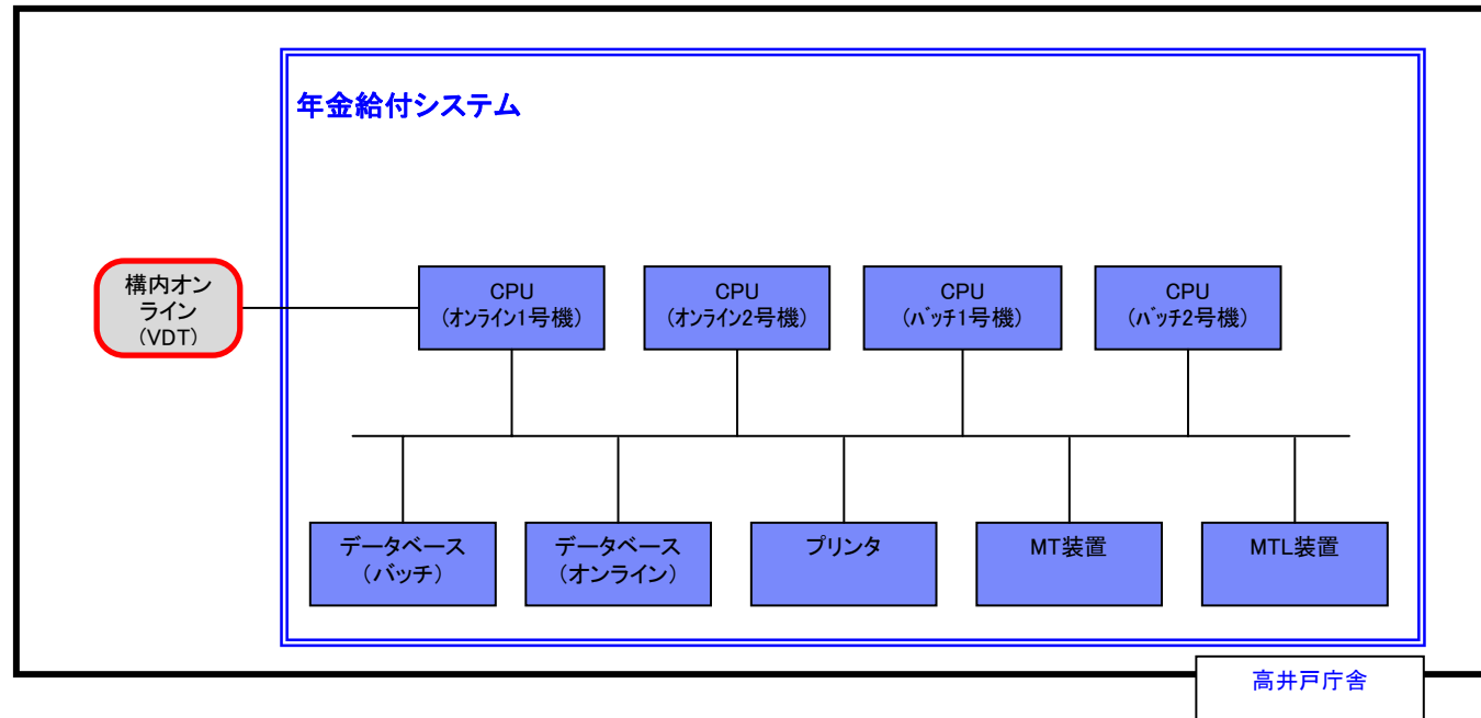
図4 ネットワーク構成図(年金給付システム)
