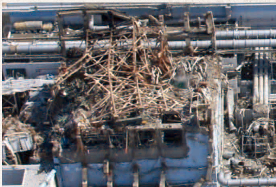
1F-3号機 原子炉建屋5階 事故直後の状況
