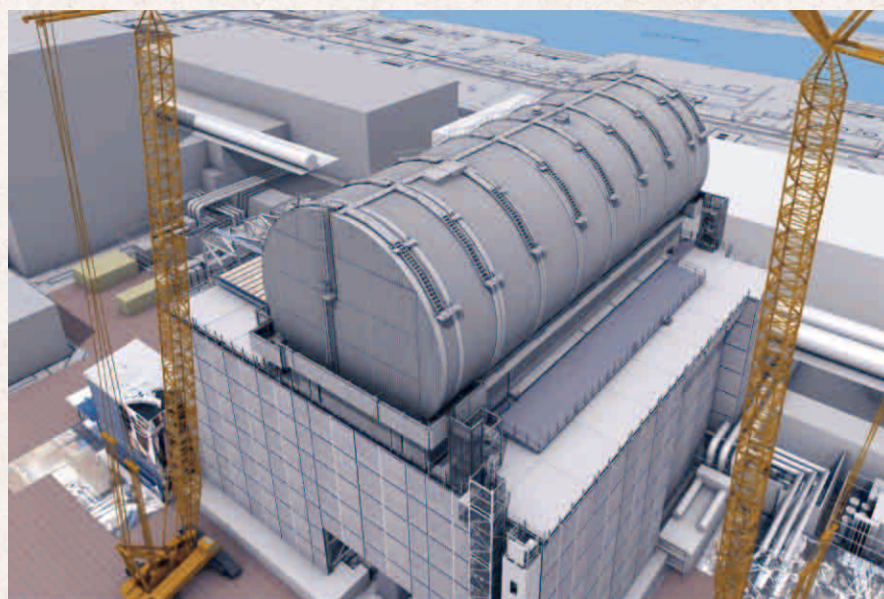
1F-3号機 原子炉建屋5階 燃料取出し用カバー設置イメージ図 資料提供:鹿島建設(株)
