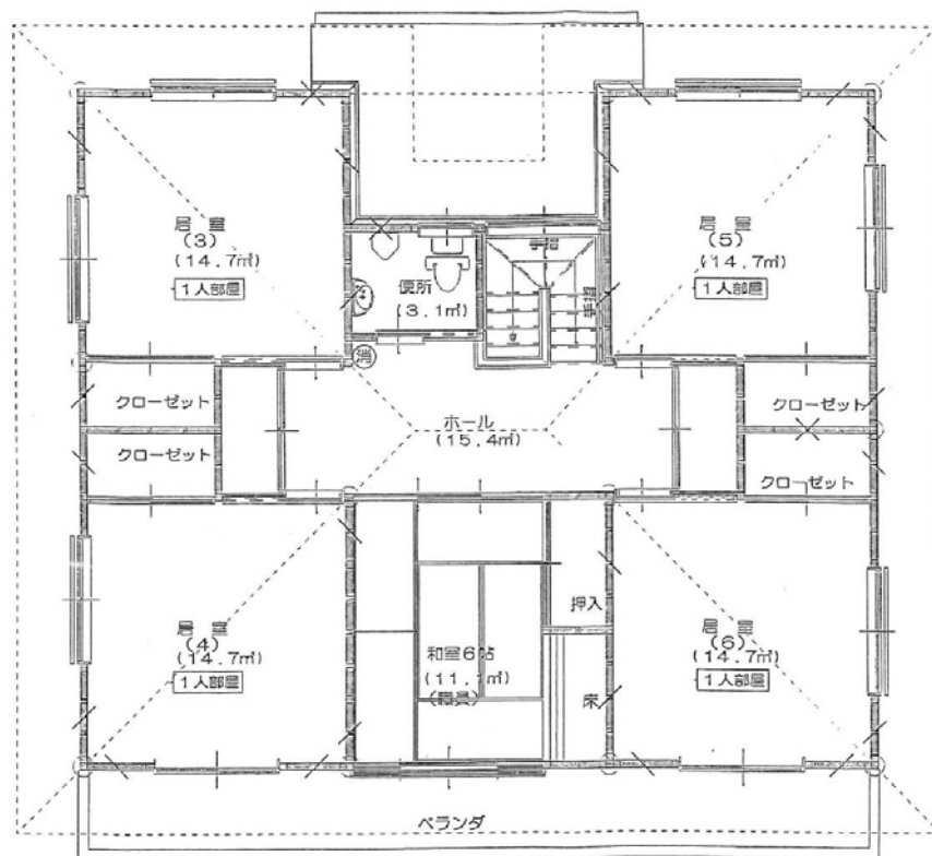
2階 平面図
