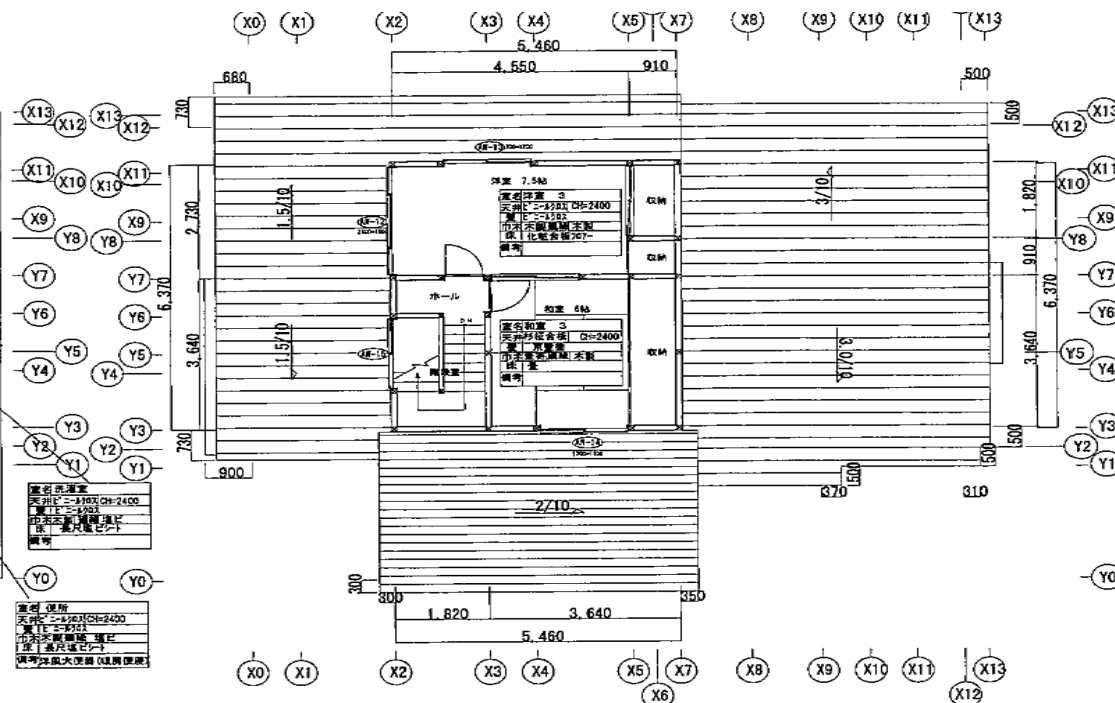
2階既存平面図 1/100
