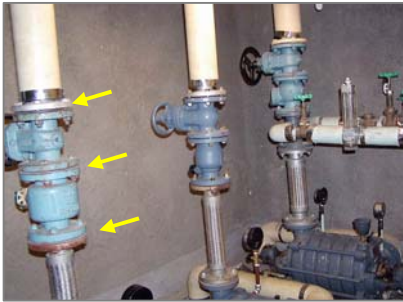
バルブ継ぎ手部などへのパッキング・ガスケット (継ぎ目に挟まっていますので写真では見え ていません)
