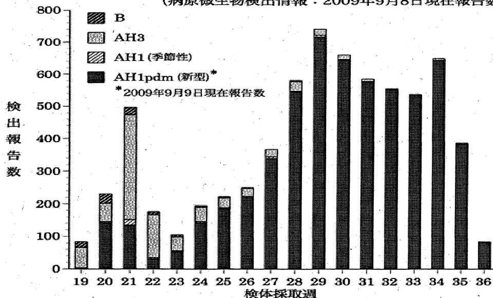
週別インフルエンザウイルス分離・検出報告数、2009年第19～36週 （病原微生物検出情報：2009年9月8日現在報告数）
