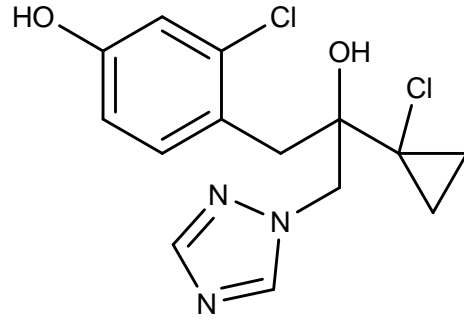
代謝物 M21
