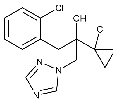
代謝物 M17
