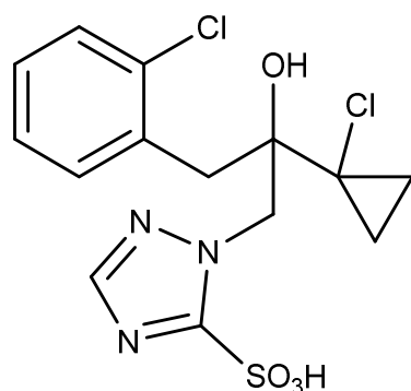
代謝物 M07
