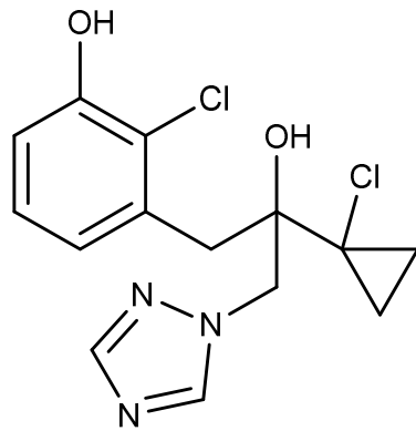
代謝物 M20
