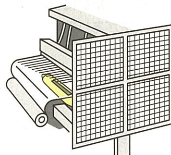
シャトルガードの設置例
