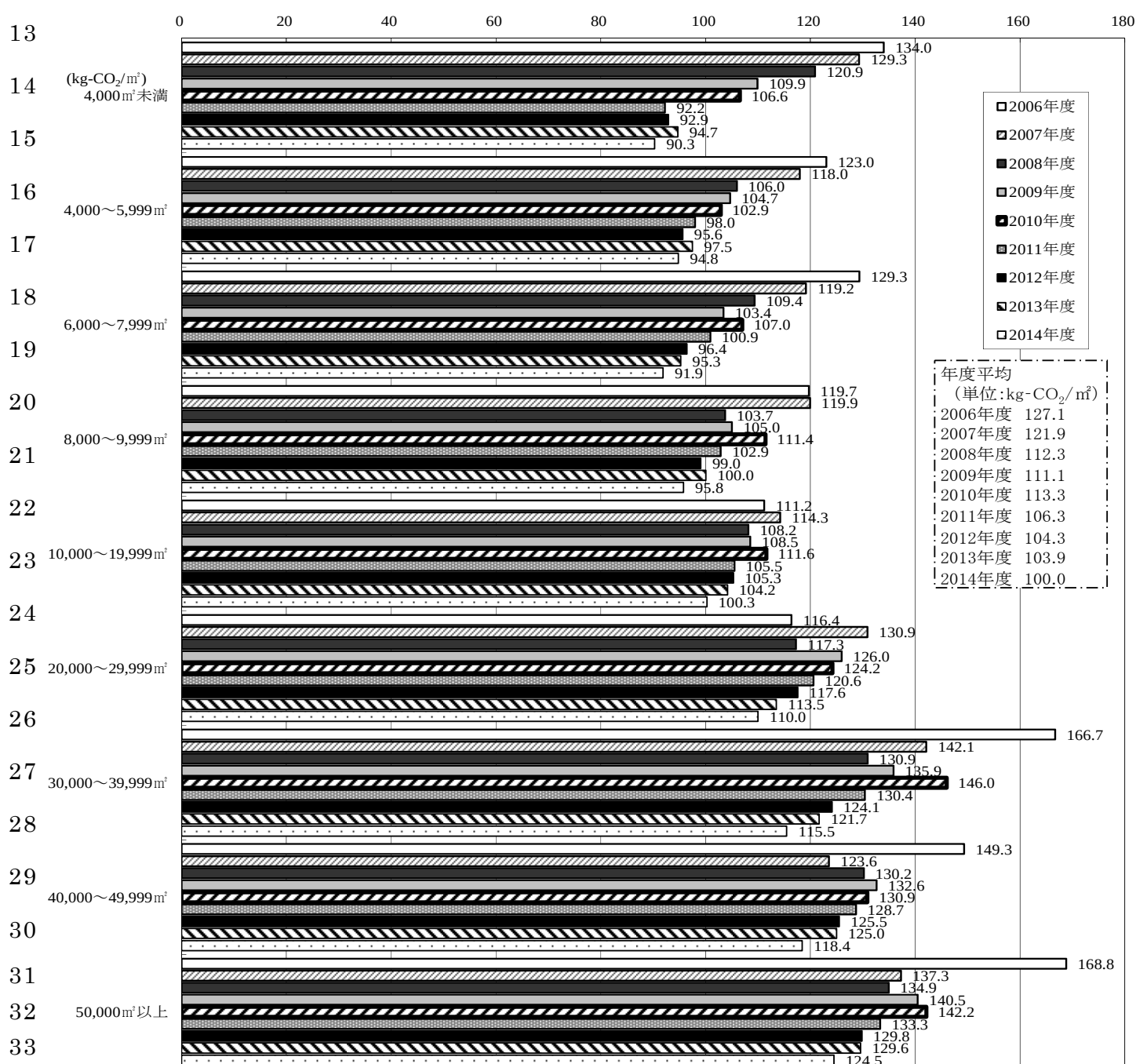
12 図4-1 病院規模別（延べ床面積規模別）のCO 2 排出原単位の推移
