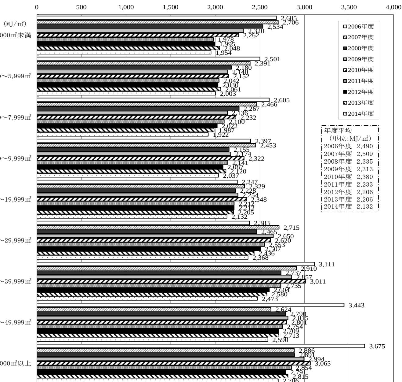
図4-2 病院規模別(延べ床面積規模別)エネルギー消費原単位の推移
