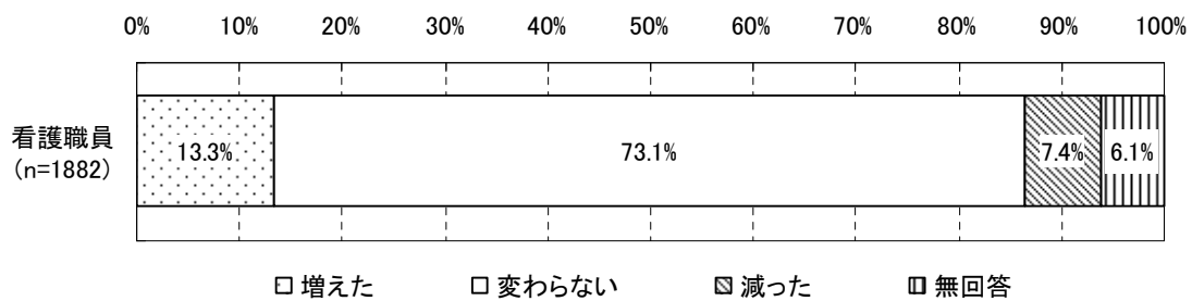
図表 346 夜勤時の受け持ち患者数
