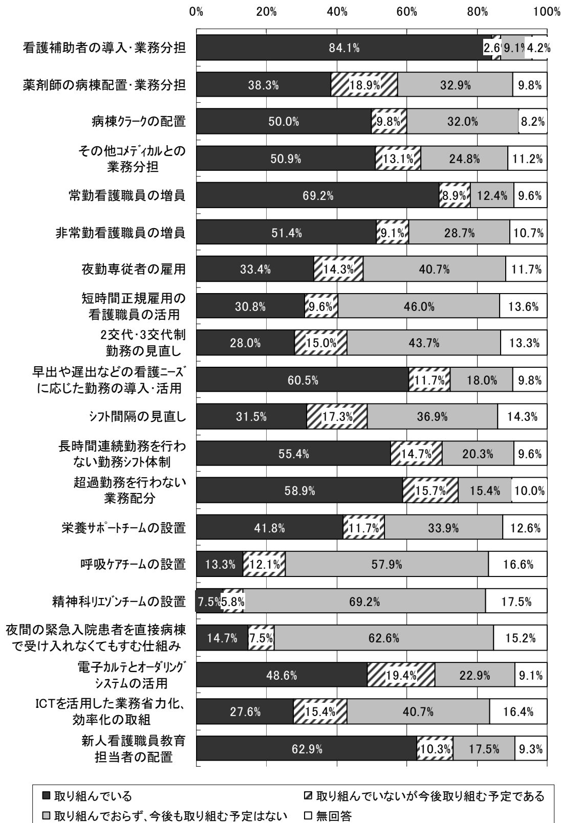
図表 194 看護職員の負担軽減策の取組状況 (n=456)
