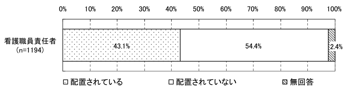
図表 324 病棟への薬剤師の配置状況
