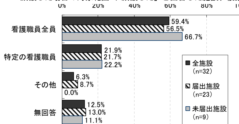
図表 159 減額した場合の対象範囲（「減額した」と回答した施設、複数回答）
