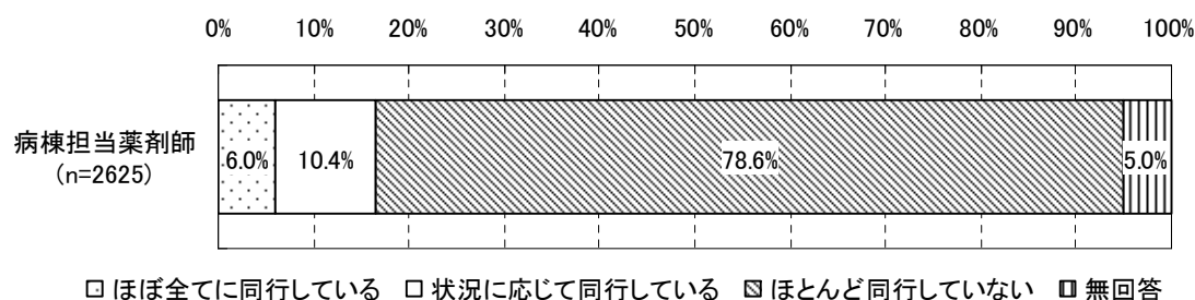
図表 398 医師の回診への薬剤師の同行
