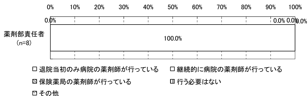
図表 383 在宅患者訪問薬剤管理指導等の状況 (在宅患者訪問薬剤管理指導料等を算定している施設)
