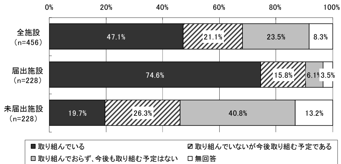
図表 186 勤務医の負担軽減策の取組状況 ～⑫電子カルテとオーダリングシステムの活用～
