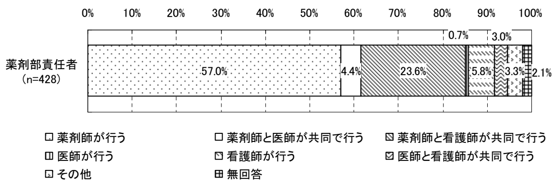
図表 373 入院患者が持参した薬の確認状況
