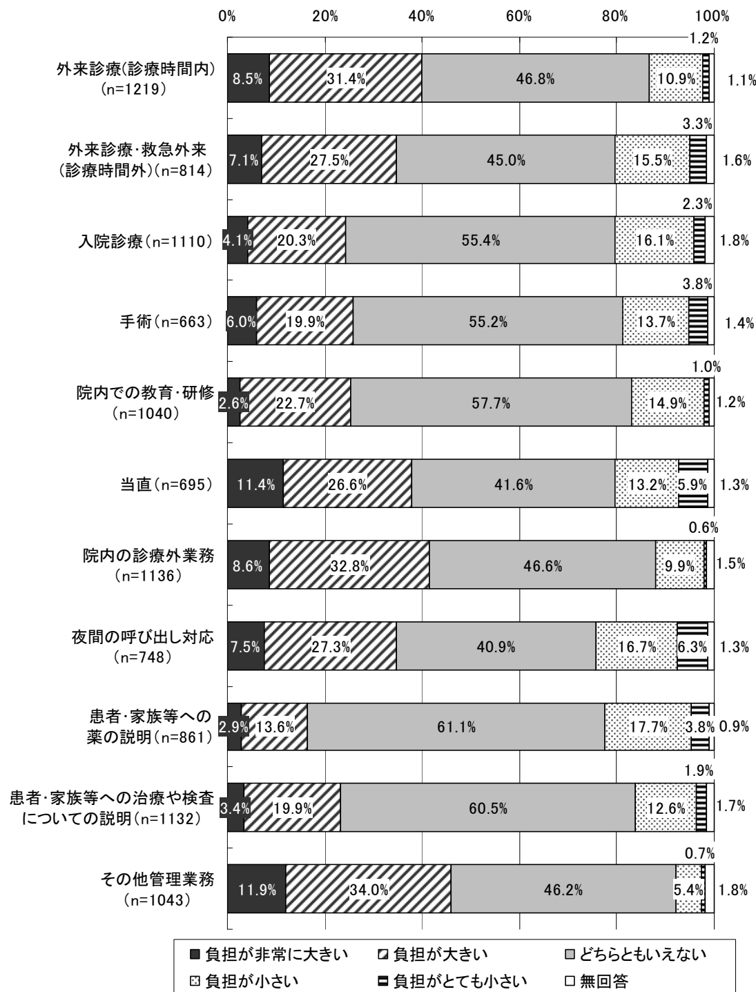
図表 251 担当している業務の負担感（各業務を行っている医師責任者）
