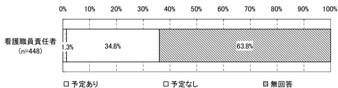
図表 306 看護補助加算の届出の予定
