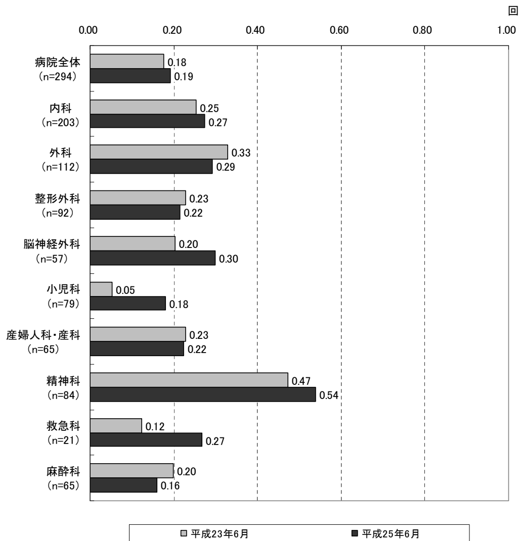
図表 123 医師 1 人あたりの連続当直回数（1 か月分、非常勤医師（常勤換算）） ＜全施設＞
