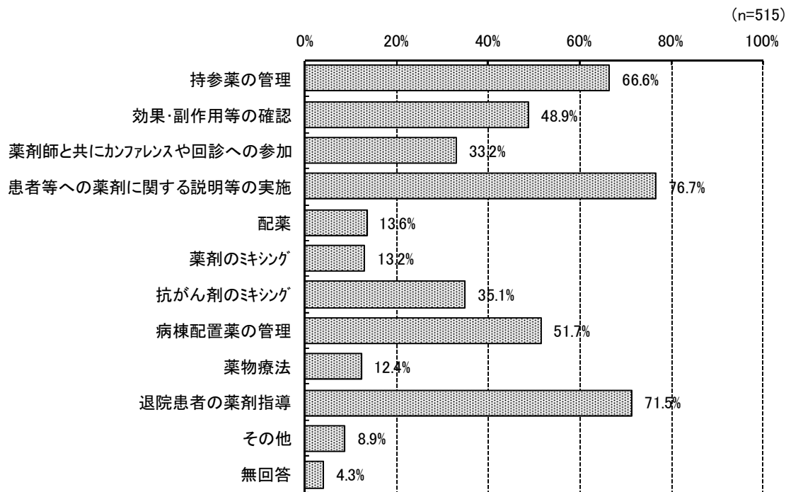
図表 325 病棟薬剤師との連携内容 (薬剤師が配置されている病棟、複数回答)
