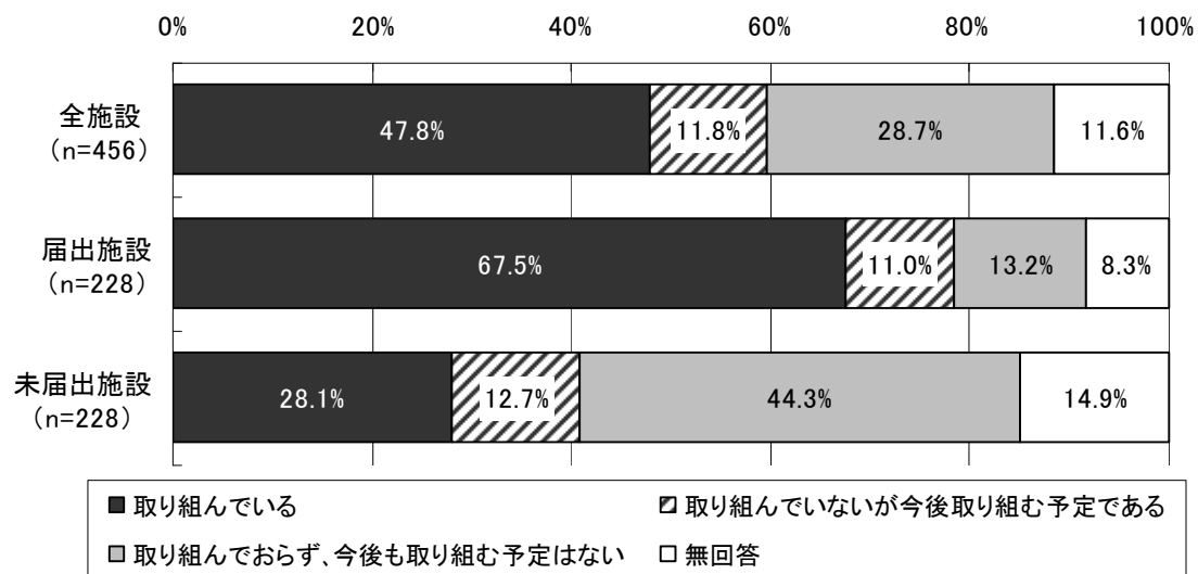
図表 177 勤務医の負担軽減策の取組状況
