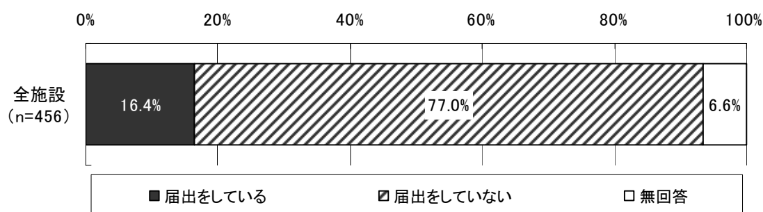
図表 205 移植後患者指導管理料の施設基準の届出
