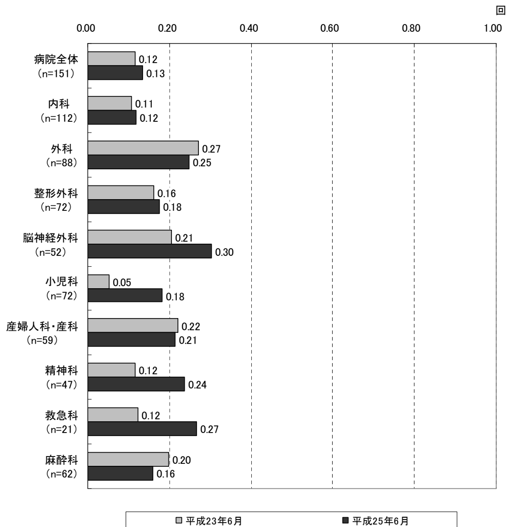
図表 124 医師 1 人あたりの連続当直回数（1 か月分、非常勤医師（常勤換算）） ＜届出施設＞
