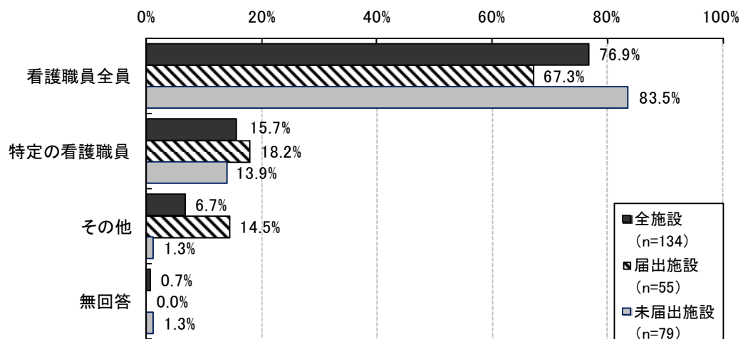
図表 155 増額した場合の対象範囲（「増額した」と回答した施設、複数回答）
