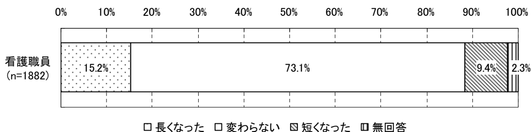
図表 342 長時間連続勤務の状況
