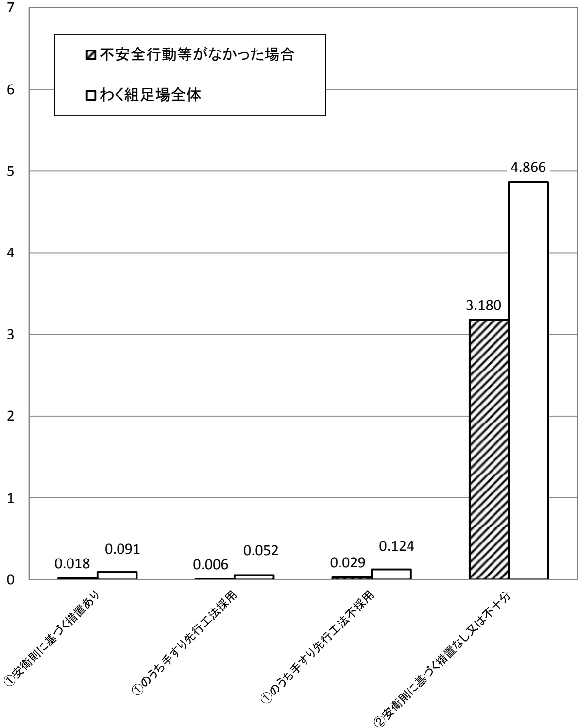
わく組足場1000現場当たりの墜落災害発生件数(推計)
