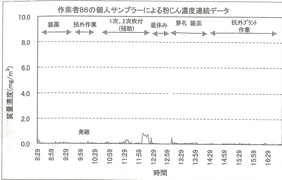
図 12 作業者B6 じん質量濃度連続データ
