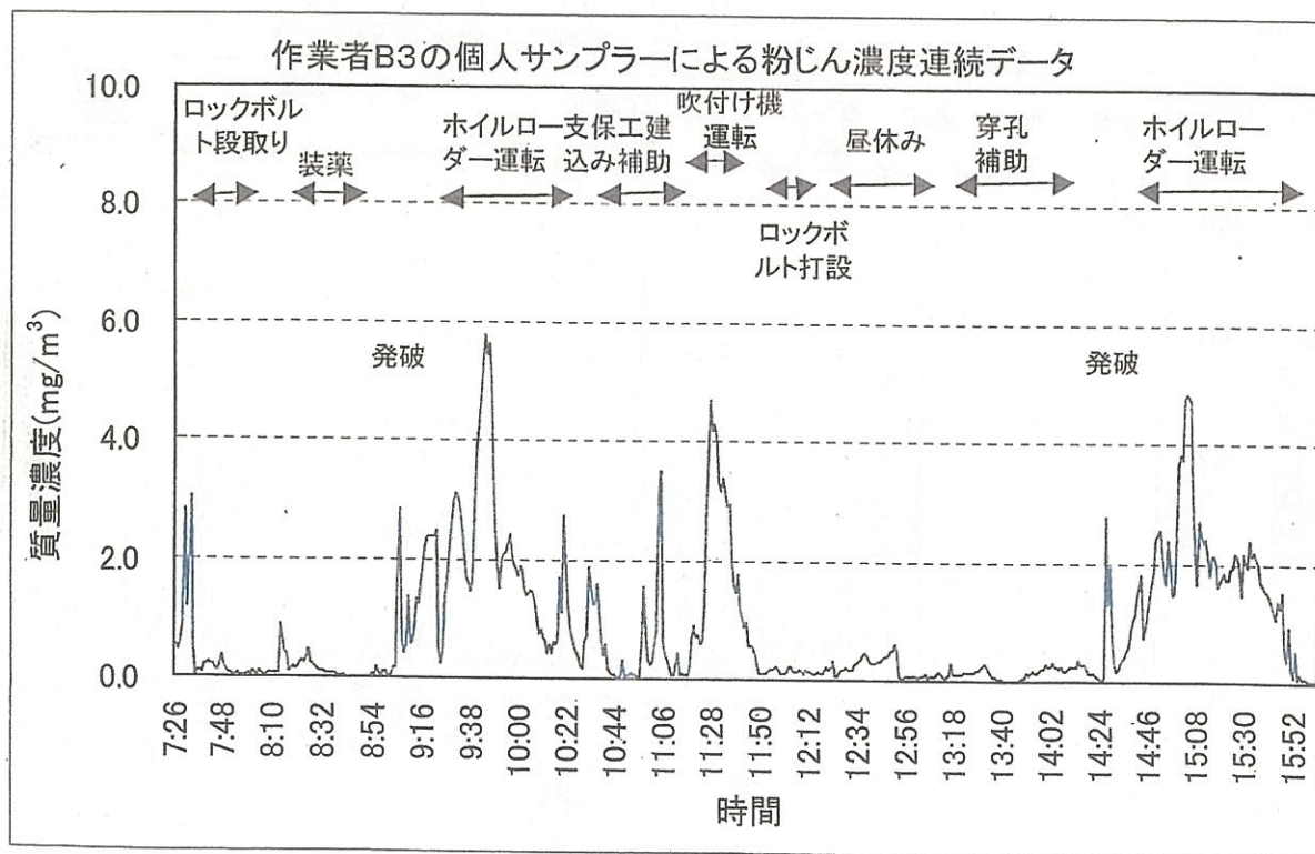
図 9 作業員B3の粉じん質量濃度連続データ
