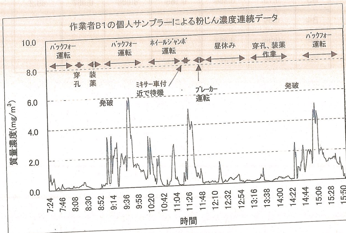
図 7 作業員 B 1 の粉じん質量濃度連続データ
