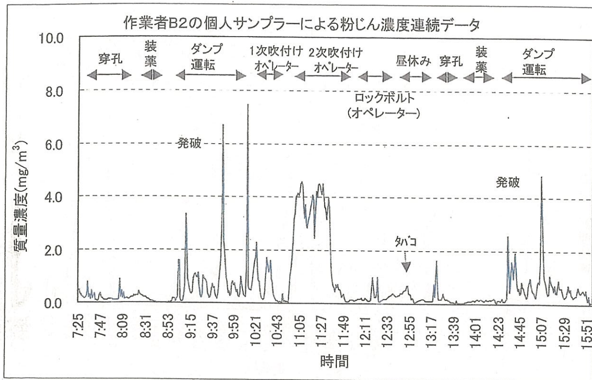
図 8 作業員B2の粉じん質量濃度連続データ
