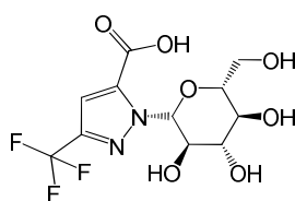
代謝物 Z
