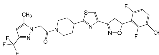
代謝物 L
