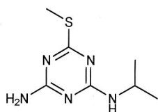
代謝物B
