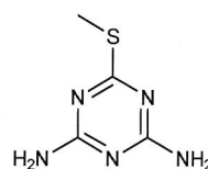
代謝物C
