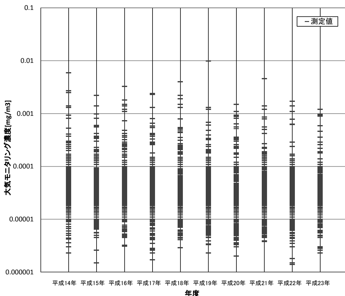
図 5-1 クロロエチレンの過去 10 年間の年度別大気環境モニタリング調査結果のプロット図
