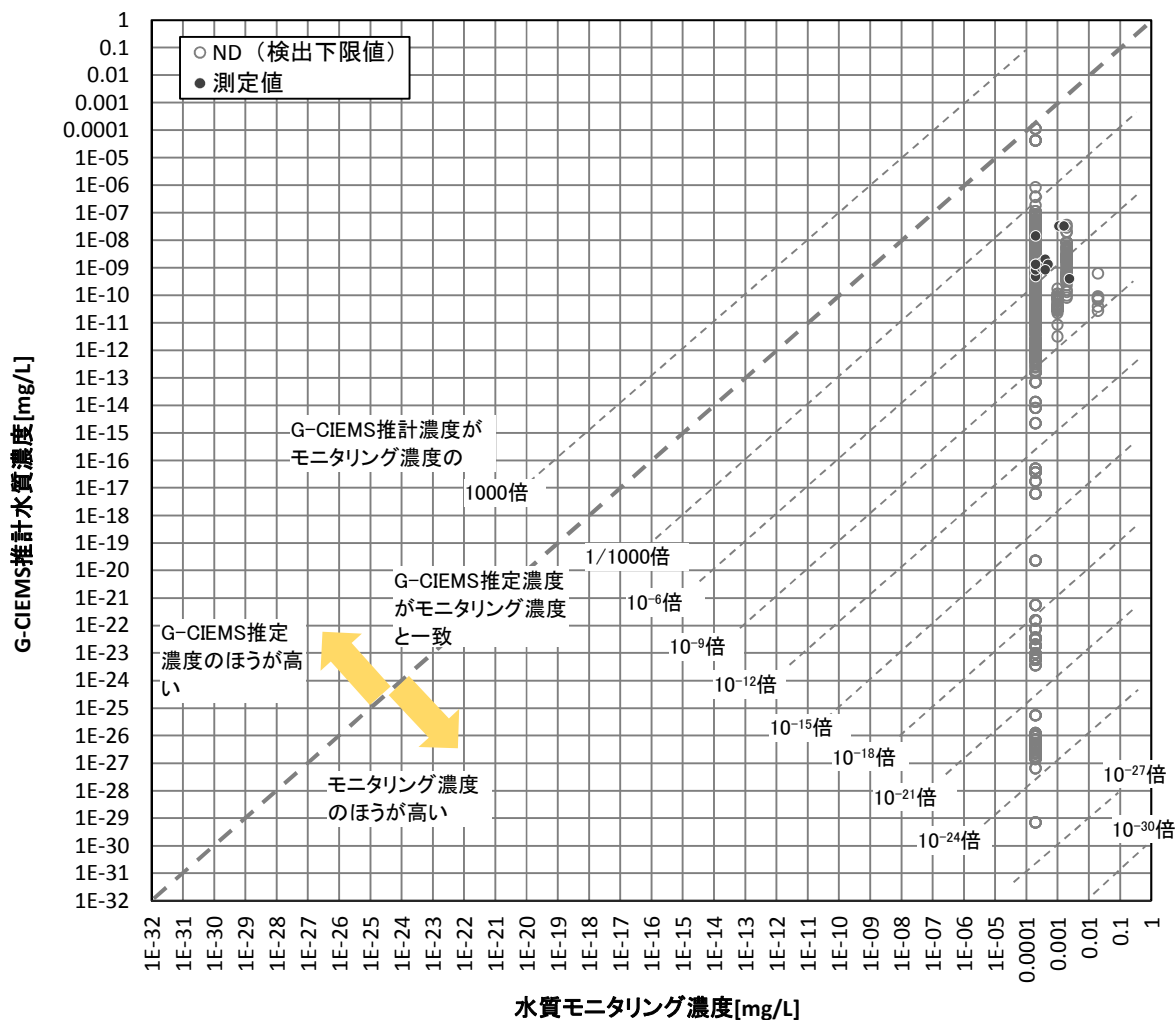
図7-3 評価対象地点のG-CIEMS推計水質濃度とモニタリング水質濃度の比較(要監視項目(平成19～23年度))
