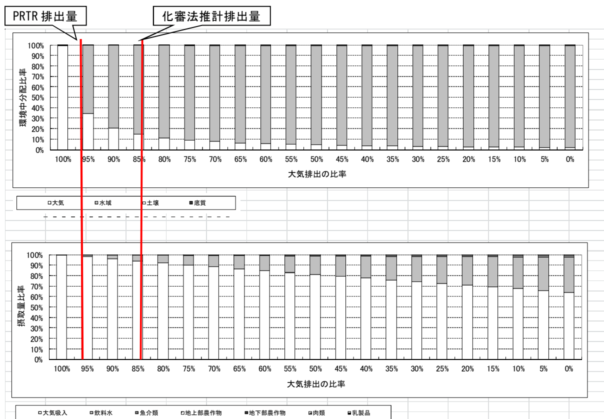
図 5-7 排出先比率の変化による環境中分配比率と摂取量比率の変化
