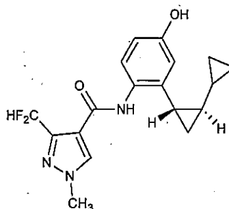
代謝物 E
