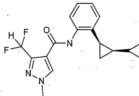
cis 体
