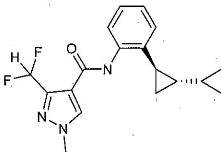
trans 体
