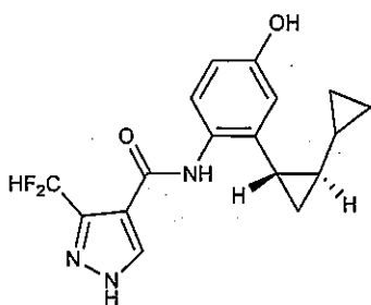
代謝物 B
