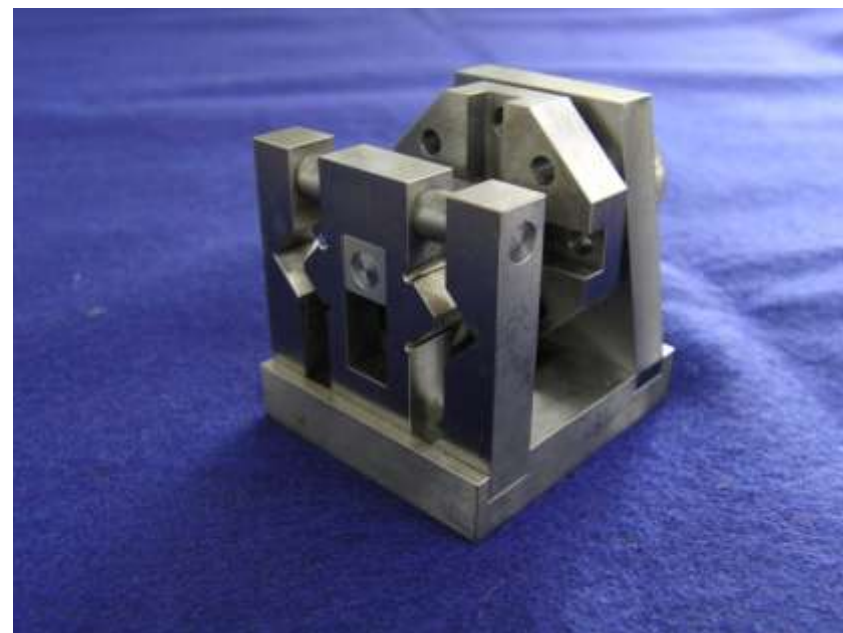
マルチプルランメルギヤ機構倍速装置
