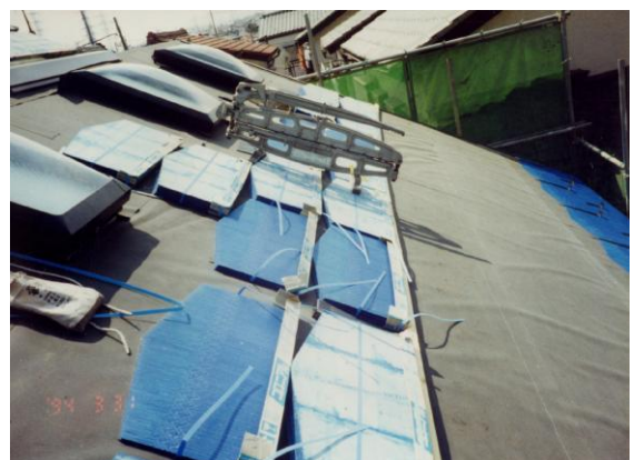
図 2.35 石綿含有ルーフィングの施工例
