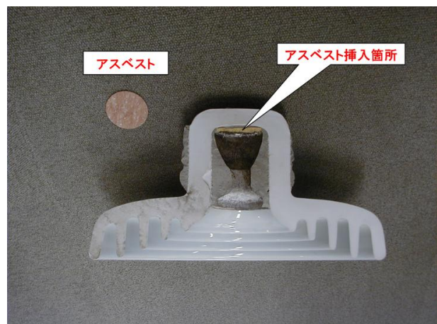
図 2.54 緩衝材（送電）
