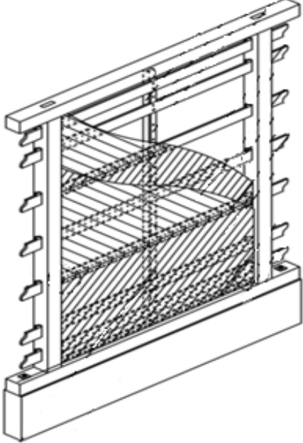
耐震壁の構造
