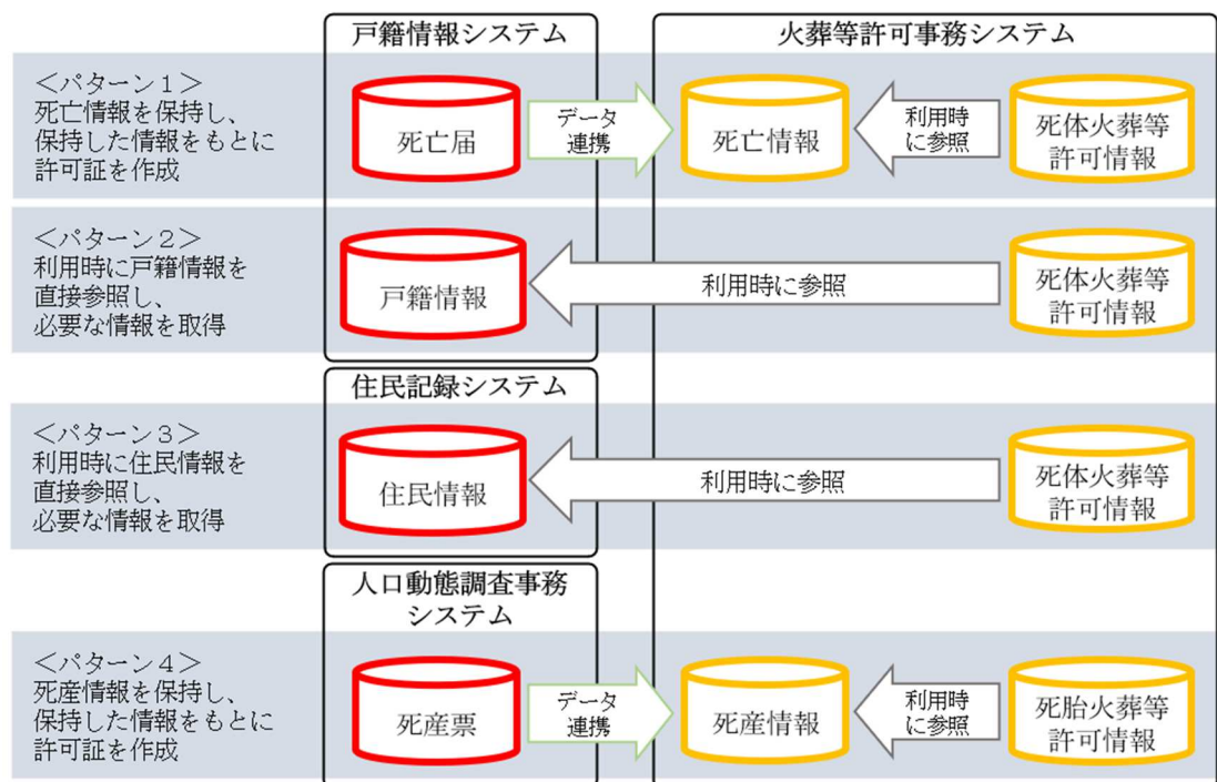
図 3-3 基幹系他システムとの連携イメージ
