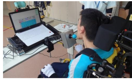
らくらくマウスにより顎でカーソルを移動し、 頭部のスイッチ(ジェリービーンスイッチ)で決 定することで、PC を操作
