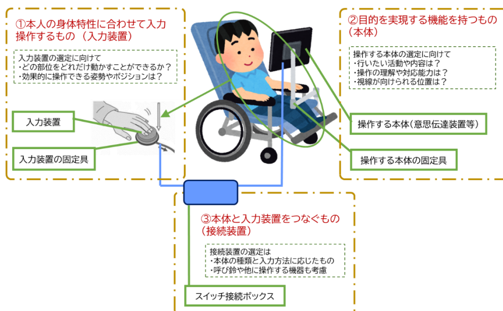
図 14 コミュニケーションのAT支援に必要な機器の構成
