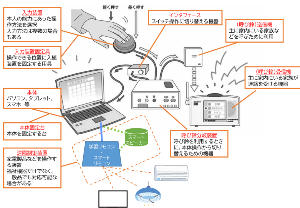
図 15 意思伝達装置の具体的構成例
