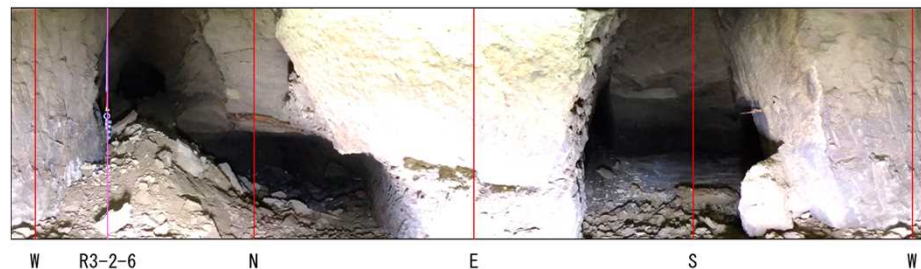
地下壕R3-2
