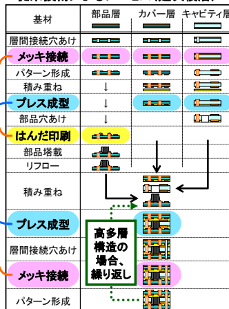
◆従来の製造プロセスとの比較 (工程数を1/3に縮減)
