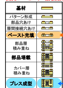
◆従来の製造プロセスとの比較 (工程数を1/3に縮減)
