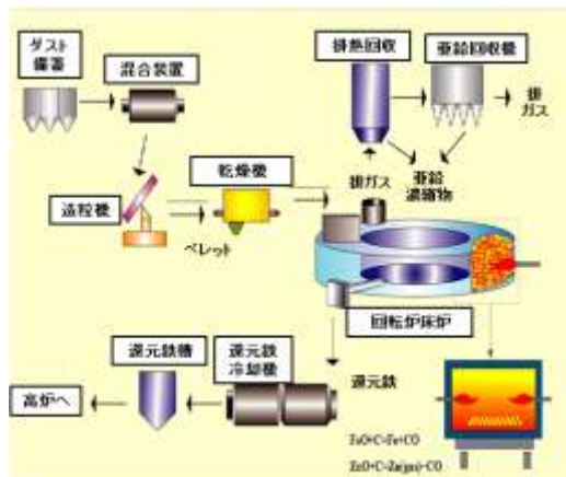
◆リサイクルプロセス全体像 (※右下のドーナツ形が「回転炉床還元炉」)
