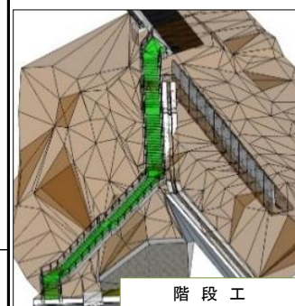
3次元モデルを用いた施工検討会 (Construction discussion using 3D model)
