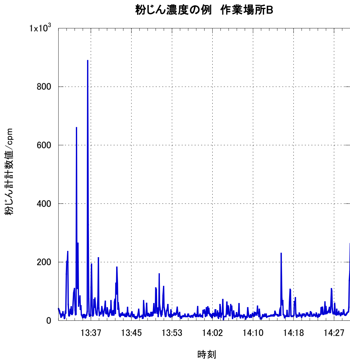
図 3 粉じん濃度の時系列変化例（2 回目調査のデータ）
