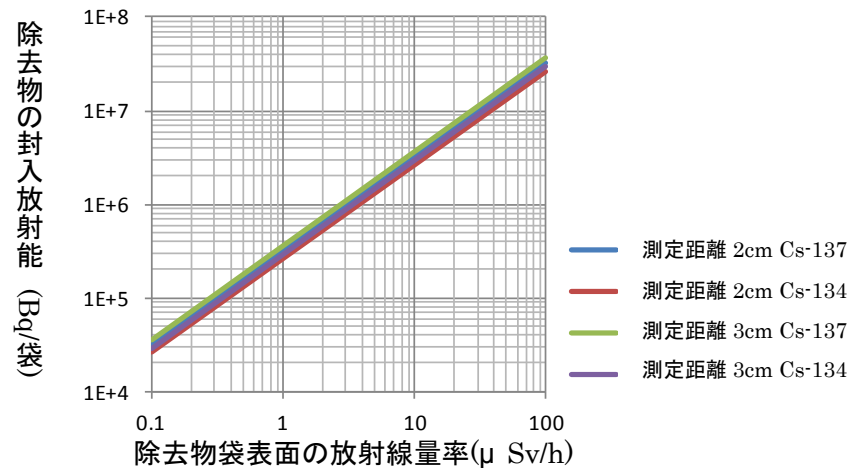
(土のう袋)
