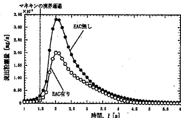
図-13 EACの有無における流出粉塵量の比較
