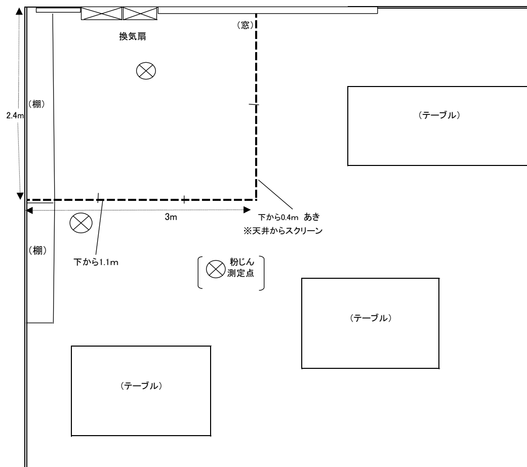
平面图
