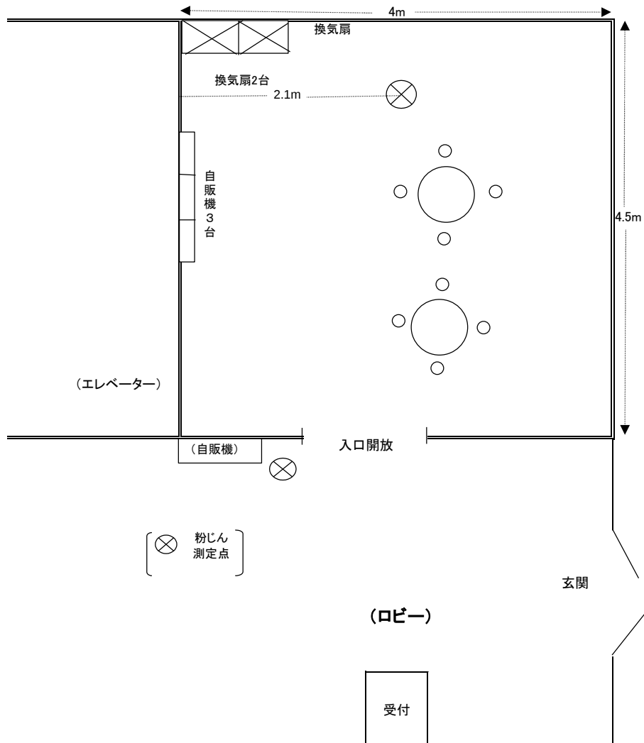
平面図
