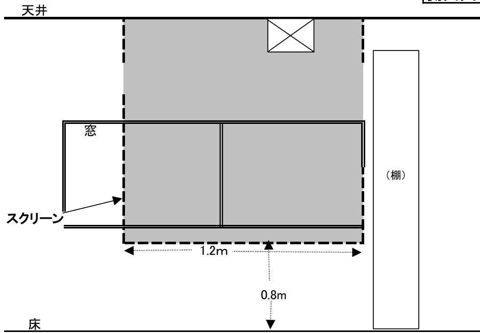
側面図
