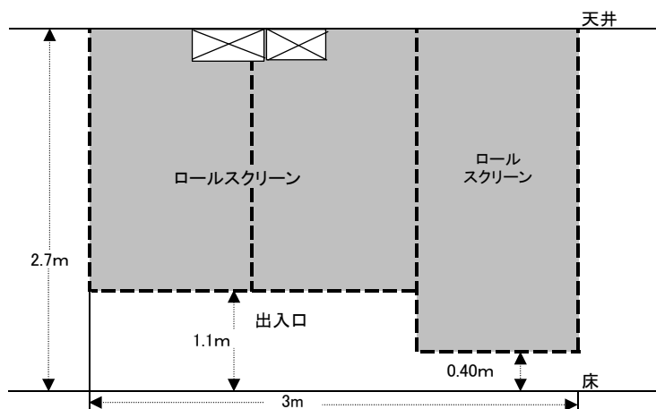
側面図
