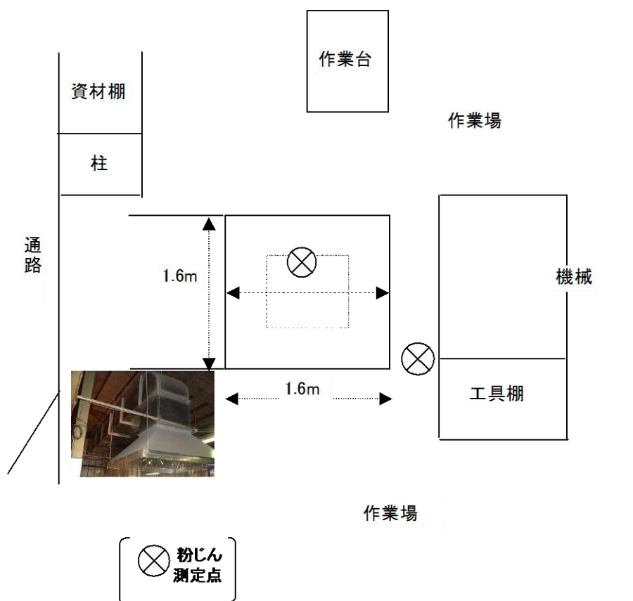
平面図
