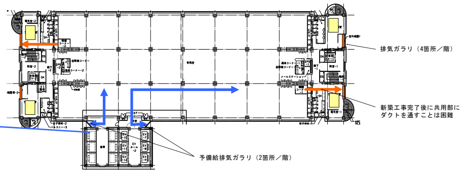
基準階平面
