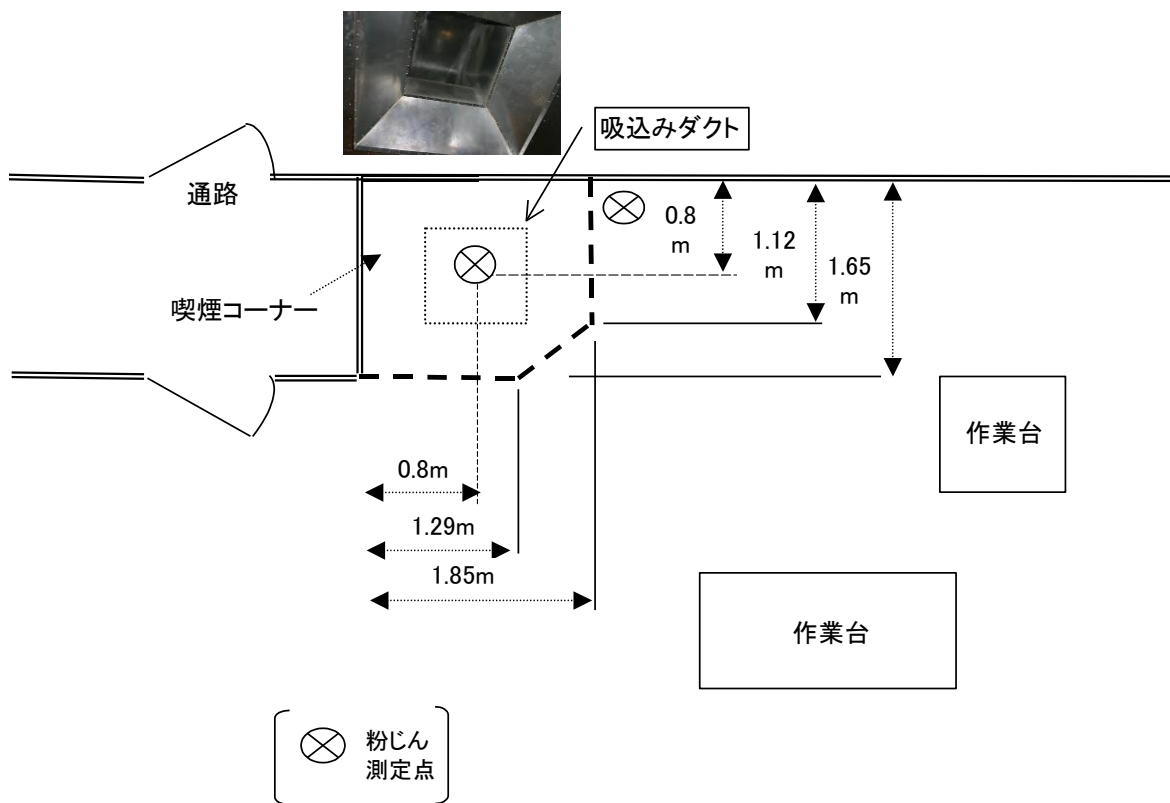
平面図
