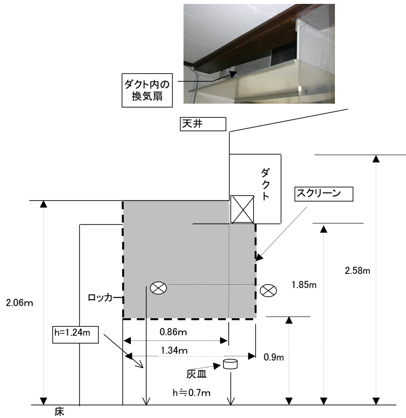
側面図
