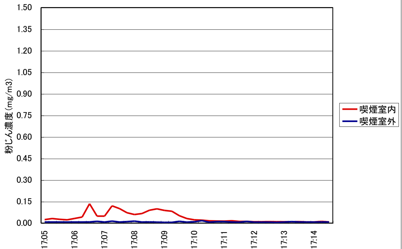
事例12 既存の建築物に設置した喫煙室
