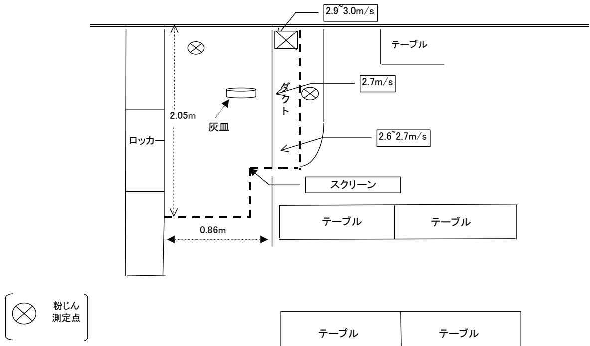
平面図
