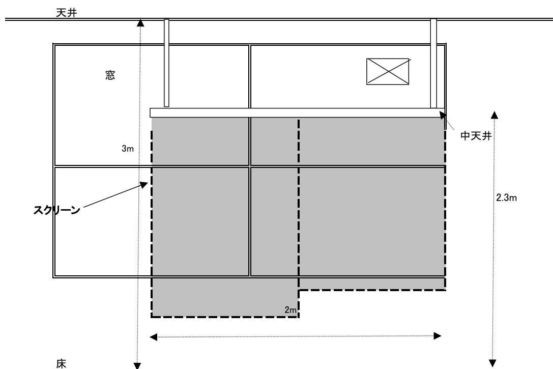
側面図
