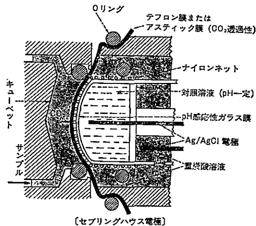
図 21 P_{CO_2} 電極
