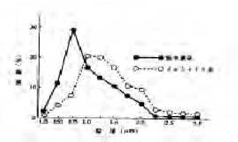
図 46 被覆アーク溶接棒ヒュームの粒度分布（一例）
