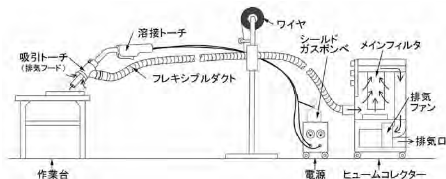
図 52 ヒューム吸引トーチの構成例
