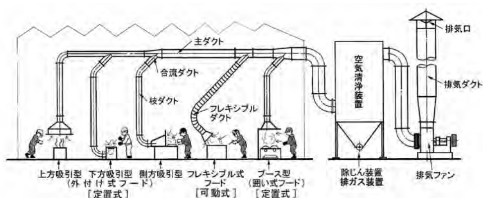
図 48 局所排気装置の構成例
