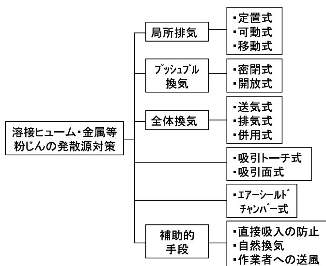
図 47 溶接ヒューム、金属等粉じんの発散源対策
