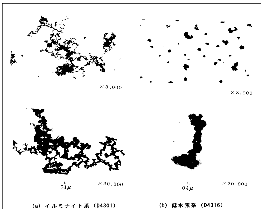
図 45 自然沈降ヒュームの電子顕微鏡写真
