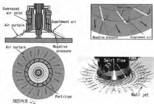
図 54 防風エアースールドチャンバー
