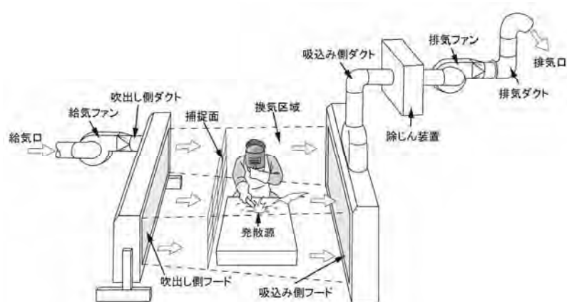
図 51 開放式プッシュプル型換気装置の構成例
