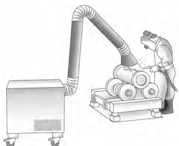
図 49 移動式局所排気装置の構成例
