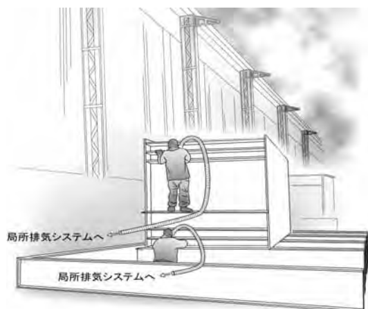
図 50-1 屋外アーク溶接作業への応用例 1
