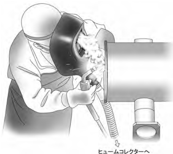
図 53 吸引溶接面を使用した事例
