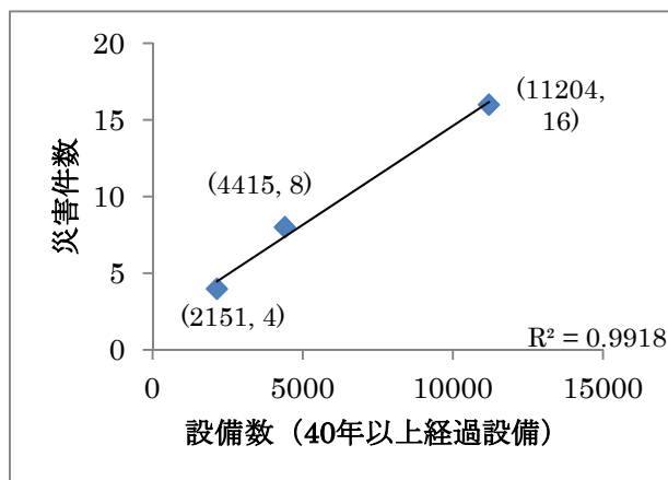
図 3 災害件数と設備数の関連 (40 年以上経過設備)
